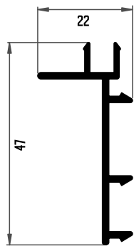
▶▶ 019 ACOPLA PARA JAMBA LISA ▶▶
