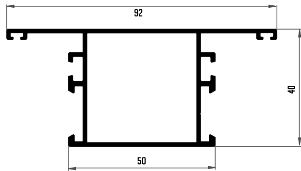
210 TRAVESAÑO PORTADA
