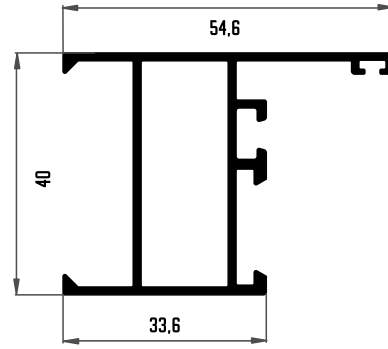
201 MARCO CON DREJAS
