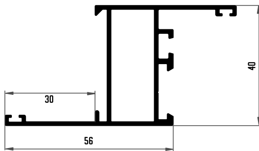
202 MARCO CON SOLAPE
