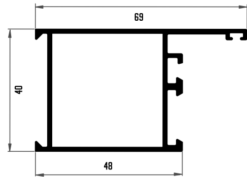
203 MARCO PORTADA
