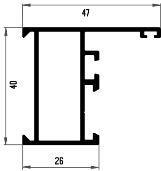
200 MARCO SIMPLE
