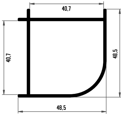
217 ESQUINERO 40 MM
