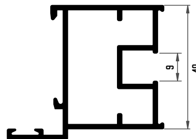
330 MARCO PARA LAMA FIJA
