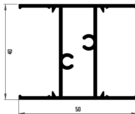
335 TRAVESAÑO CON GUSANILLO
