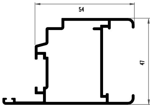
339 HOJA
