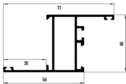
202 MARCO CON SOLAPE
