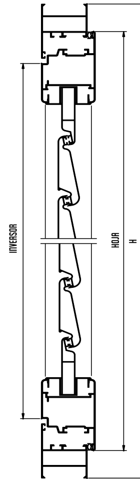
SECCIÓN B-B
