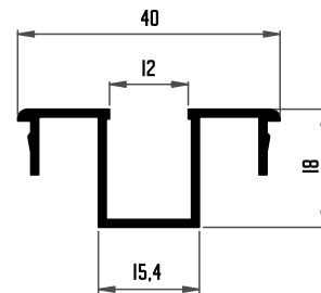
336 DIVISIÓN DE CRISTALES
