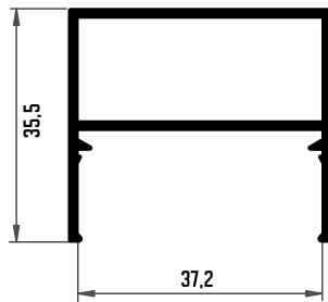
341 PERFIL MALLORQUINA
