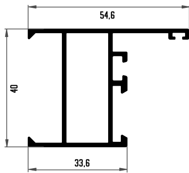
201 MARCO CON OREJAS
