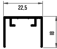
02055 MARCO/HOJA PUERTA
