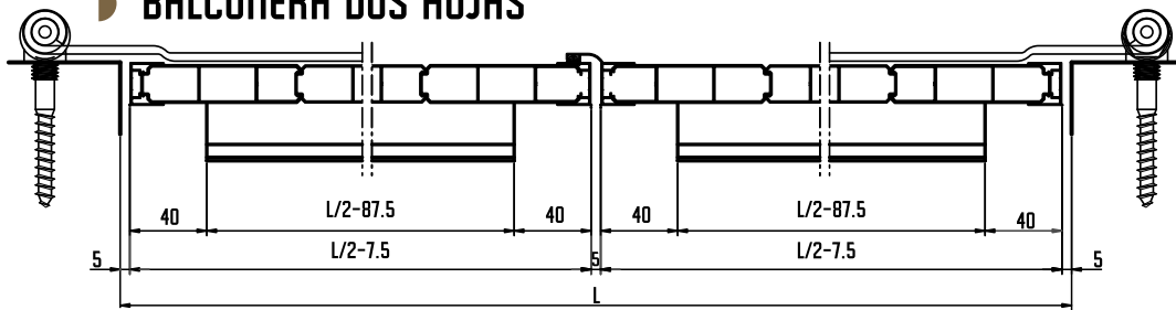
SECCIÓN A-A
