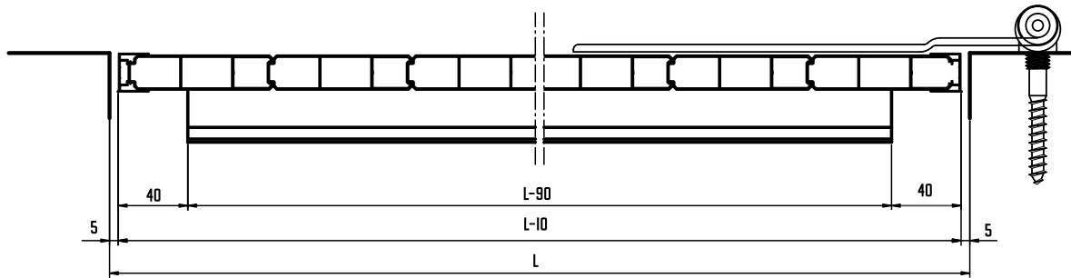
SECCIÓN A-A
