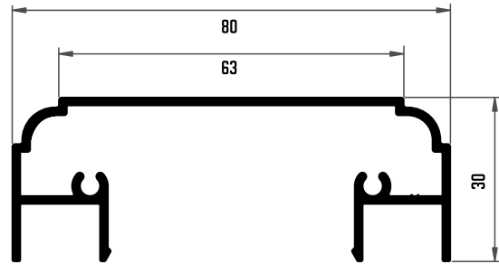
02058 TAPA HORIZONTAL
