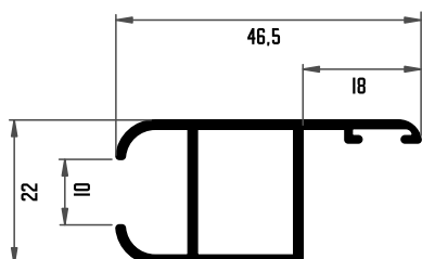
391 PERFIL DE CONTRAVENTANA
