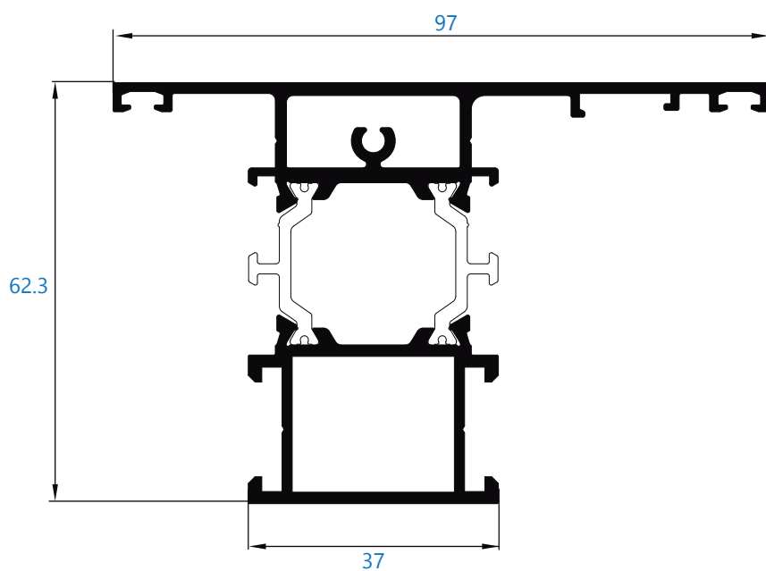
R-6261 travesaño de 97 mm
