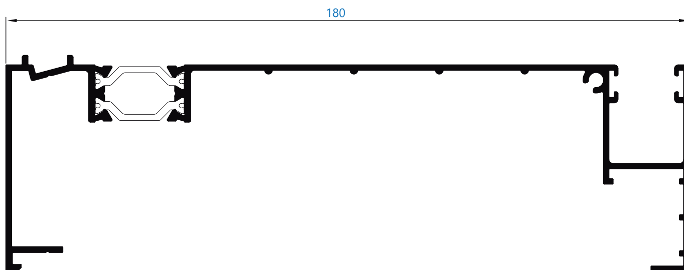
R-6587 guía de 180 mm
