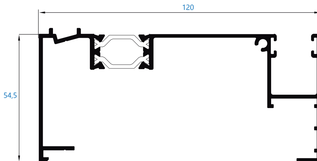
R-6589 guía de 120 mm
