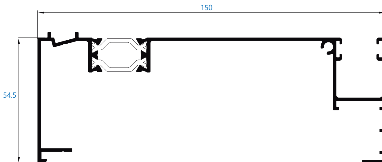
R-6288 guía de 150 mm
