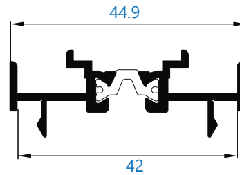
R-135 unión de cuatro hojas
