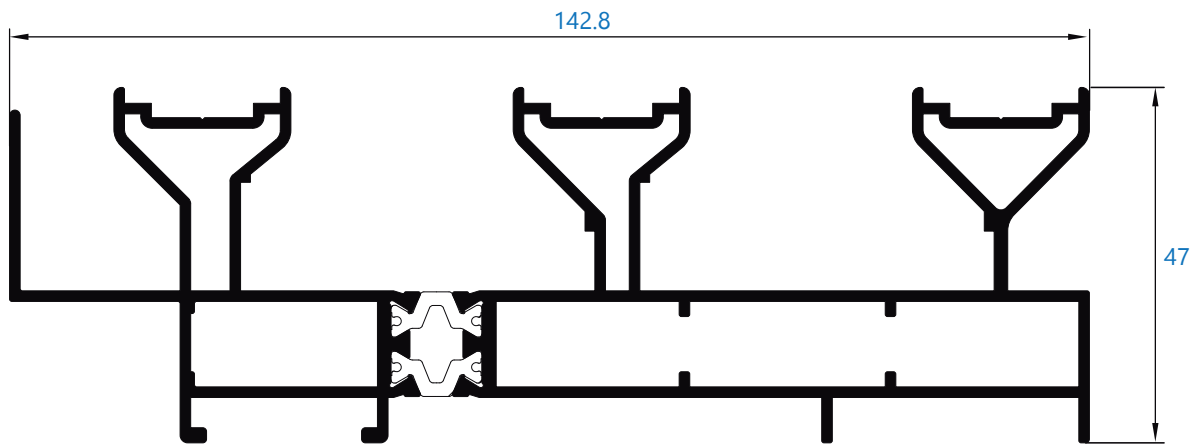
R-132 marco recto 3 carriles
