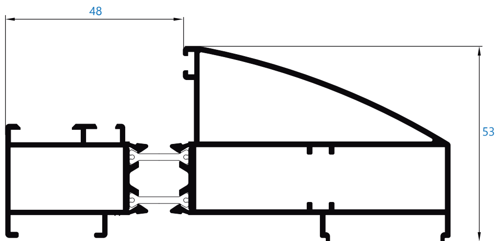
R-133 paño fijo 3 carriles
