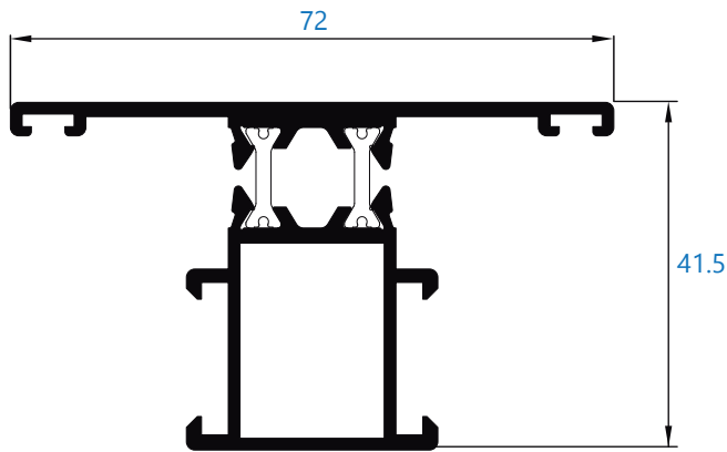
R-173 travesaño de hoja
