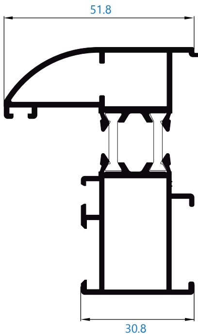
R-174 paño fijo
