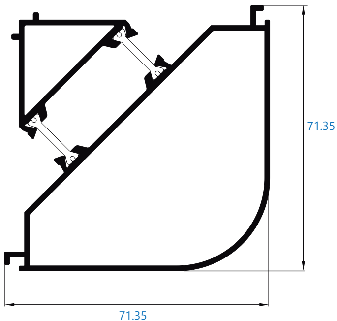
R-141 esquinero fijo
