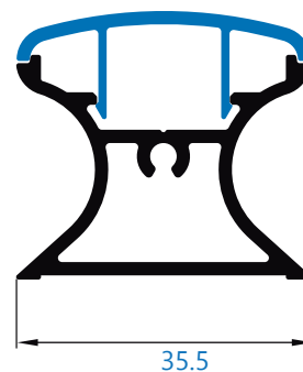
11879-80 refuerzo+tapa tirador *perfil bajo pedido
