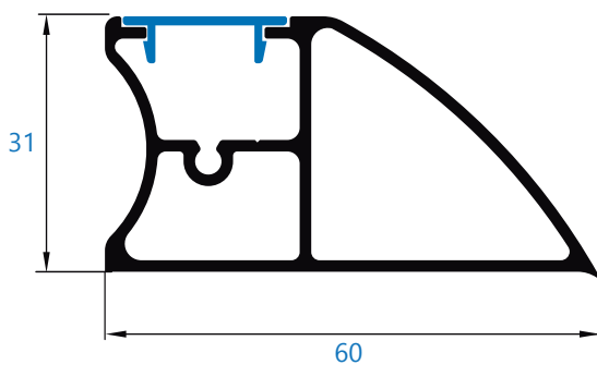
4273-77 refuerzo+tapa *perfil bajo pedido
