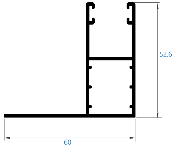
0057 guía 60 mm ala lateral *perfil bajo pedido
