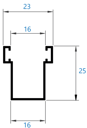
0098 guía 23 mm
