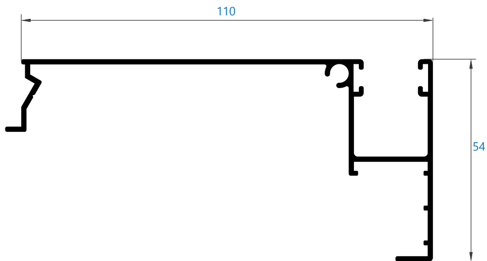
0102 guía 110 mm *perfil con pedido mínimo de kg
