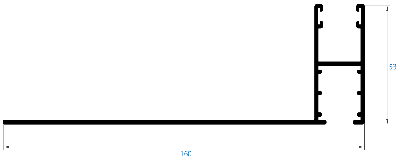
0097 guía 160 mm *perfil bajo pedido
