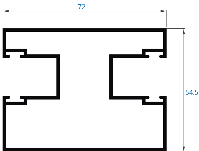
0048 guía doble polipel *perfil bajo pedido
