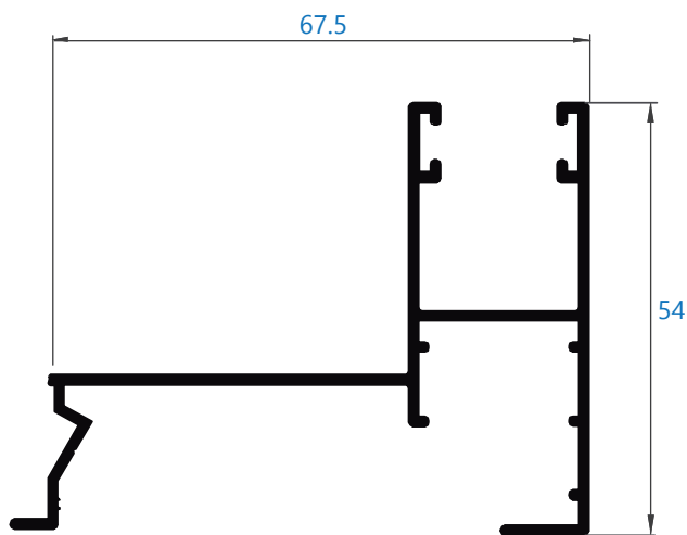
0088 guía 67,5 mm desplazada *perfil bajo pedido
