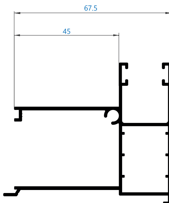
0100 guía 67,5 mm *perfil bajo pedido
