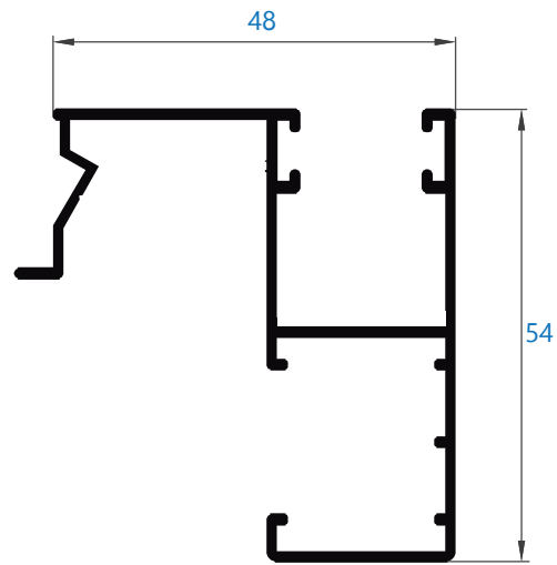
0087 guía 48 mm lateral *perfil bajo pedido
