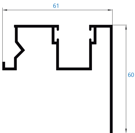
0047 guía polipel con ala *perfil bajo pedido
