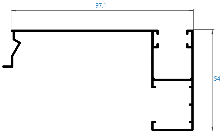
0092 guía 97,1 mm ala lateral *perfil bajo pedido
