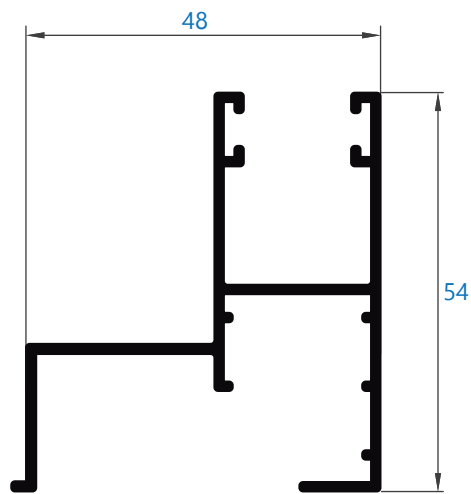
0065 guía 48 mm
