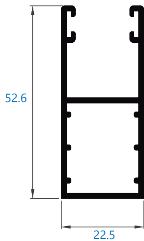
0042 guía sin aleta
