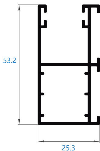
0066 guía de acople
