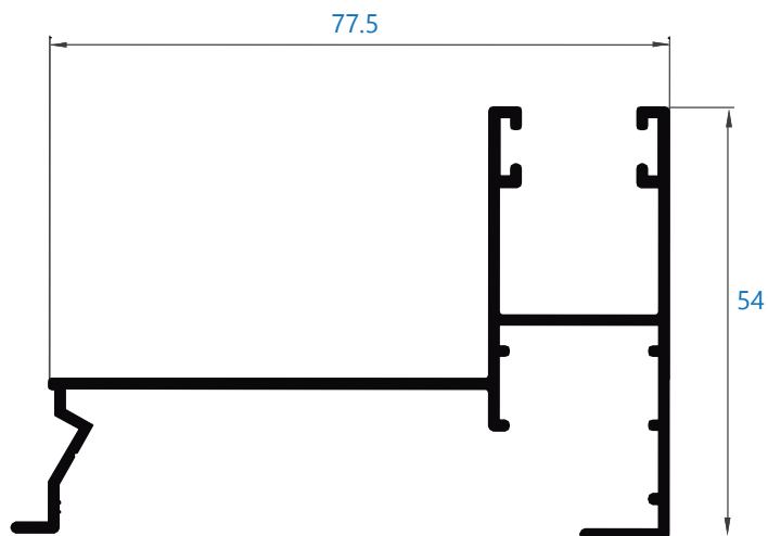
0090 guía 77,5 desplazada *perfil bajo pedido
