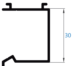
0069 acople de 30 mm
