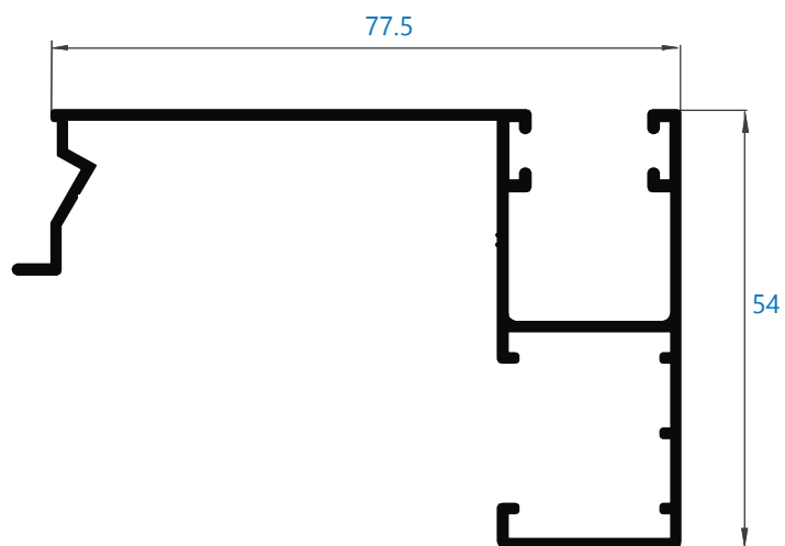
0091 guía 77,5 mm *perfil bajo pedido
