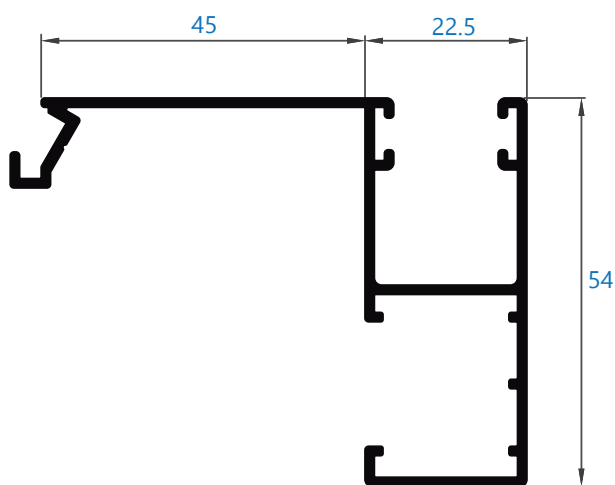
11135 guía 67,5 mm
