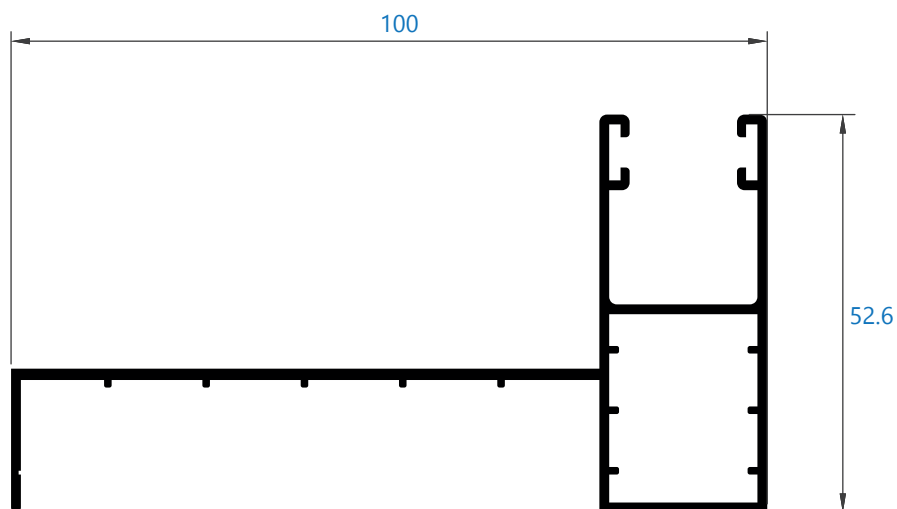
0074 guía 100 mm ala lateral desplazada *perfil bajo pedido
