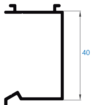
0070 acople de 40 mm
