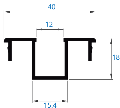
336 división de cristales
