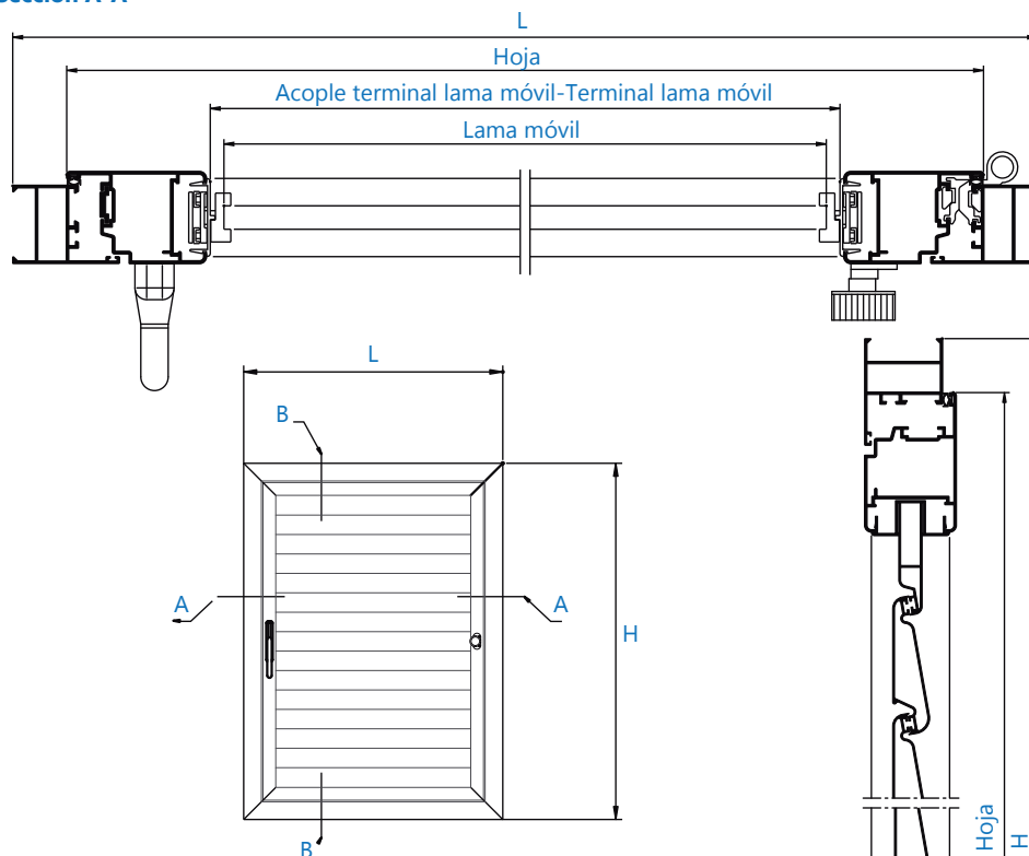
Sección A-A
