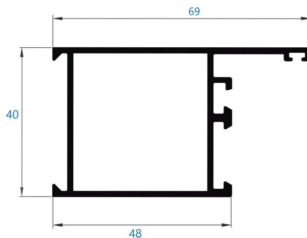
203 marco portada
