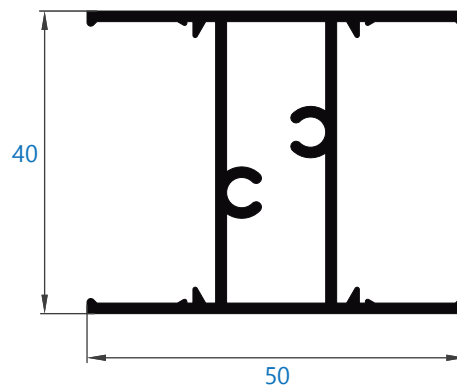
335 travesaño con gusanillo
