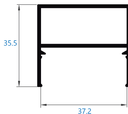
341 perfil mallorquina
