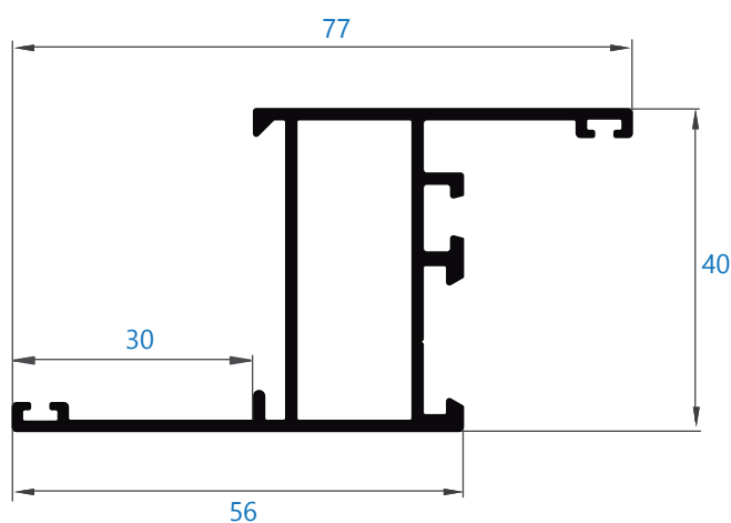
202 marco con solape
