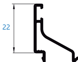
069 junquillo liso de 4 mm
