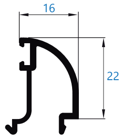
038 junquillo de 16 mm de nudo *perfil bajo pedido
