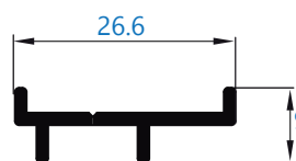
11096 suplemento de proyectante *perfil bajo pedido
