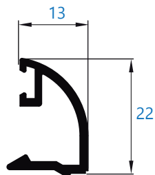
4284 junquillo curvo de 13 mm *perfil bajo pedido
