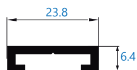
4595 suplemento de practicable *perfil bajo pedido
