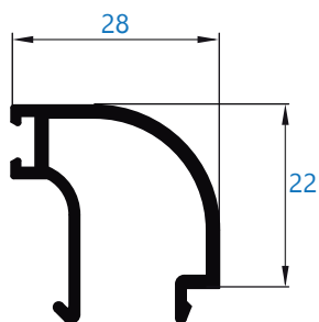
036 junquillo de 28 mm de nudo *perfil bajo pedido
