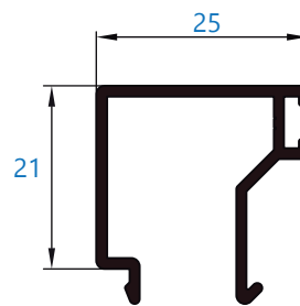
022 junquillo liso de 25 mm
