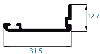
4493 solape de 31,5 mm *perfil bajo pedido
