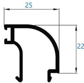
065 junquillo de 25 mm de nudo *perfil bajo pedido
