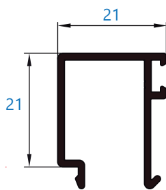
021 junquillo liso de 21 mm
