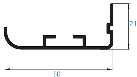
11021 solape de 50 mm *perfil bajo pedido
