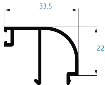
7505 junquillo de 33,5 mm de nudo *perfil bajo pedido
