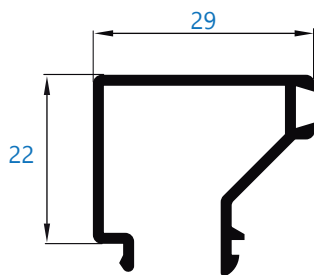
053 junquillo liso de 29 mm
