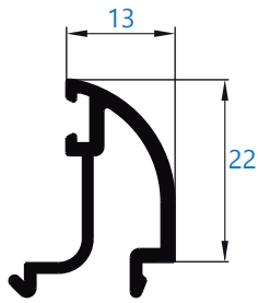
7637 junquillo de 13 mm de nudo *perfil bajo pedido
