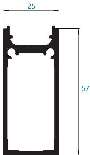
13268 refuerzo de 60 mm *perfil bajo pedido
