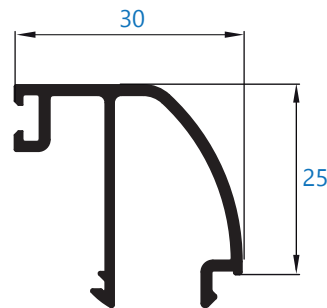
10425 junquilo de 30 mm
