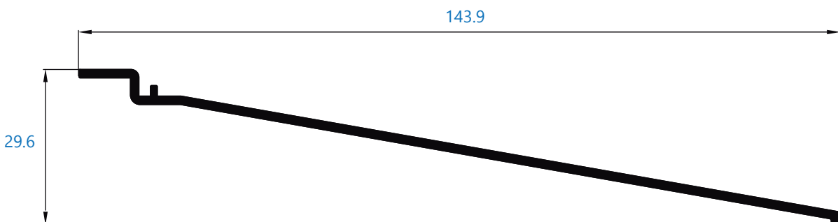
13578 alargadera de 124,5 mm
