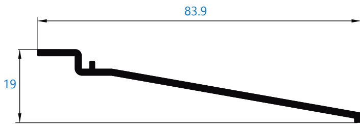
13575 alargadera de 64,5 mm
