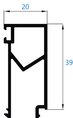
10146 junquillo de 20 mm
