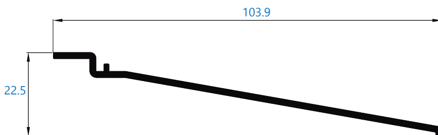
13576 alargadera de 84,5 mm
