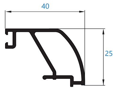
10443 junquilo de 40 mm
