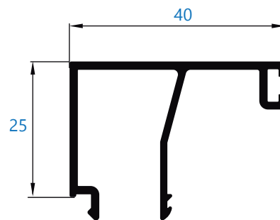
10497 junquillo de 40 mm
