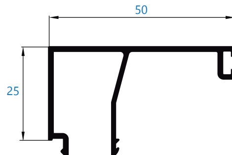
10481 junquillo de 50 mm
