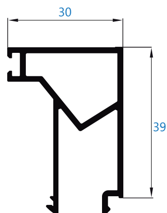
10147 junquillo de 30 mm
