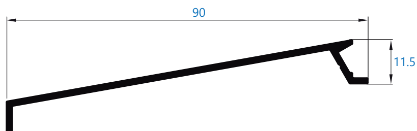
57471 goterón de 90 mm
