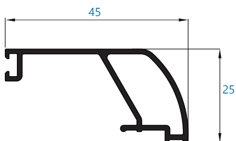
10449 junquilo de 45 mm
