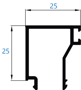
10494 junquillo de 25 mm
