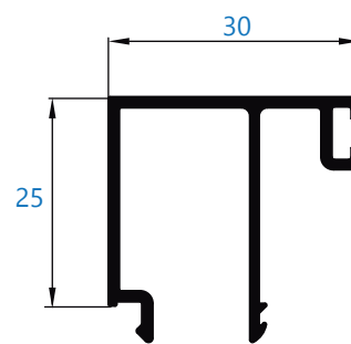
10495 junquillo de 30 mm
