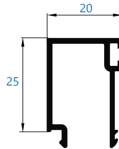
10493 junquillo de 20 mm
