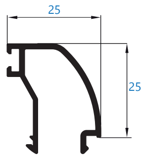
10111 junquilo de 25 mm
