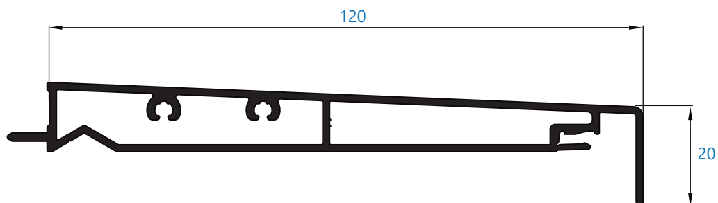
10109 alargadera de 120 mm para marco clip
