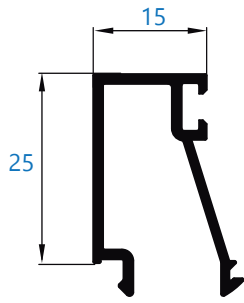
12654 junquillo de 15 mm
