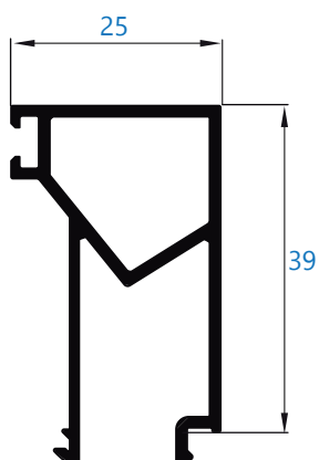
10144 junquillo de 25 mm
