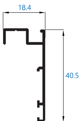
11367 solape de 40,5 mm
