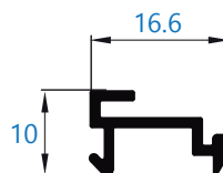
10465 acople de junquillo
