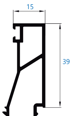
10145 junquillo de 15 mm
