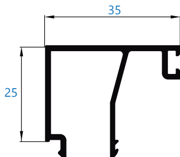
10496 junquillo de 35 mm
