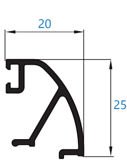
10423 junquilo de 20 mm
