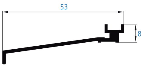
102 alargadera de 53 mm
