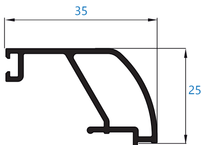
10426 junquilo de 35 mm
