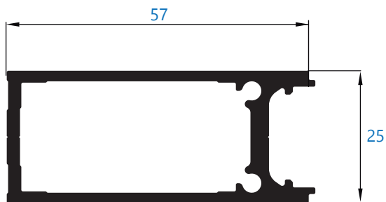
13268 refuerzo de 60 mm
