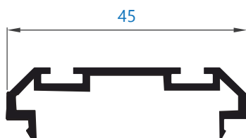
3012 acople para puerta tejana
