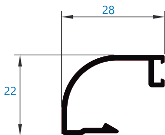
026 junquillo curvo 28 mm grapa
