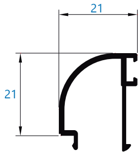
029 junquillo curvo 21 mm nudo
