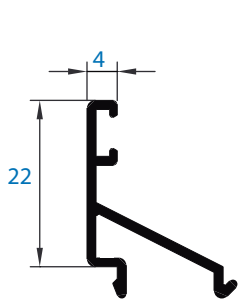
069 junquillo liso 4 mm
