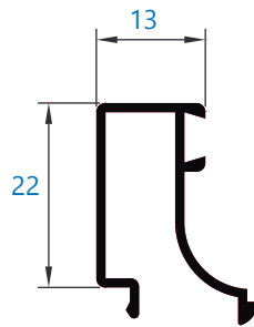
020 junquillo liso 13 mm
