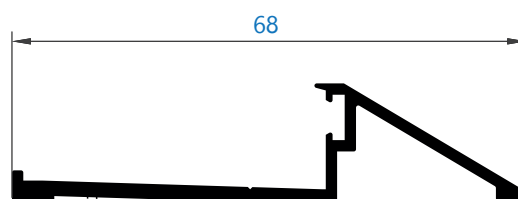
117 perfil bajo puerta *perfil bajo pedido
