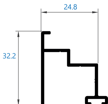
109 cortavientos puerta *perfil bajo pedido
