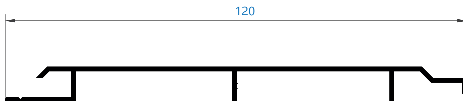
073 friso liso 120 mm *perfil bajo pedido
