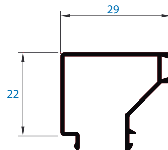
053 junquillo liso 29 mm
