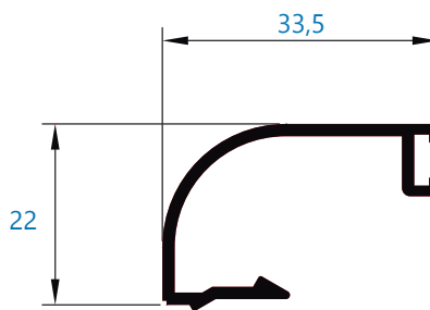
027 junquillo curvo 33,5 mm grapa
