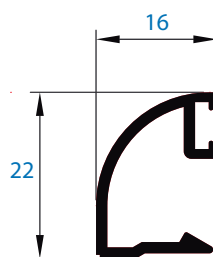
024 junquillo curvo 16 mm grapa
