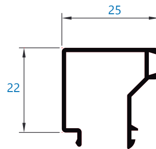
022 junquillo liso 25 mm
