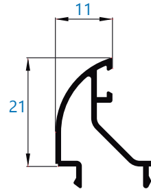
032 junquillo 11 mm retestar
