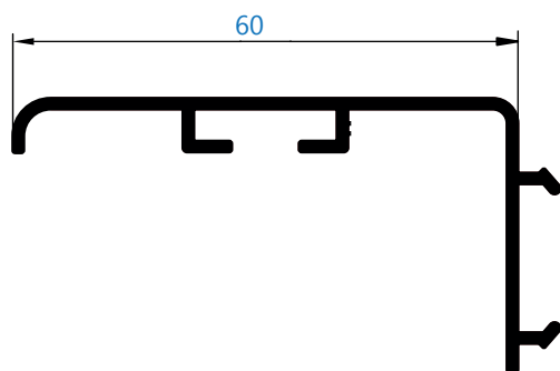
113 solape clip 60 mm *perfil bajo pedido
