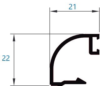
025 junquillo curvo 21 mm grapa
