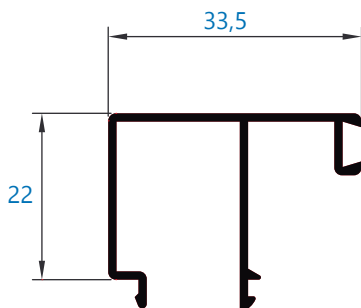
023 junquillo liso 33,5 mm
