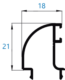
033 junquillo 18 mm retestar
