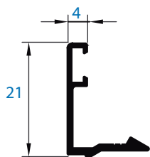
13603 junquillo liso 4 mm grapa
