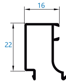
016 junquillo liso 16 mm *perfil bajo pedido
