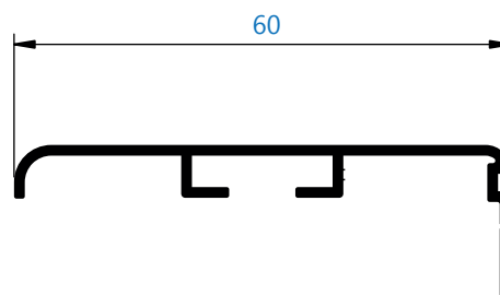
114 solape 60 mm *perfil bajo pedido
