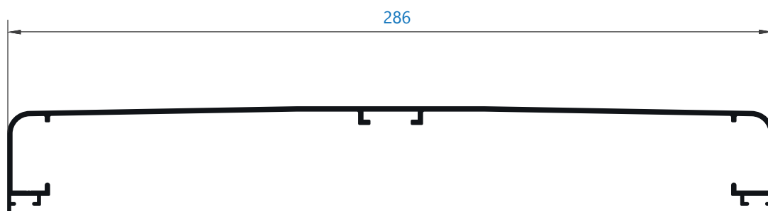
108 albardilla 286 mm *perfil bajo pedido escala 1/2
