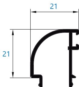
030 junquillo 21 mm retestar
