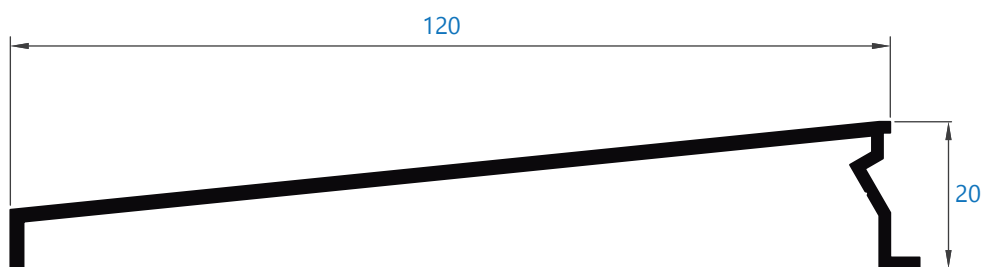
084 goterón 120 mm *perfil bajo pedido
