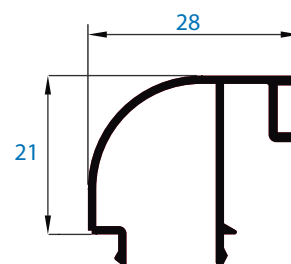
063 junquillo 28 mm retestar
