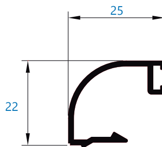
028 junquillo curvo 25 mm grapa
